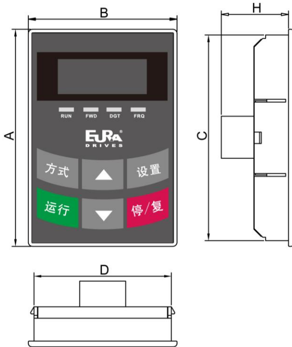
图 1-2 控制面板结构示意图
