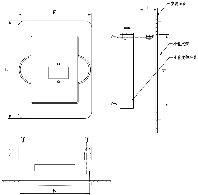
图 1-3 控制面板安装支架结构尺寸示意图
