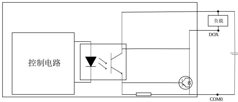
DO 输出通道电气原理图：
