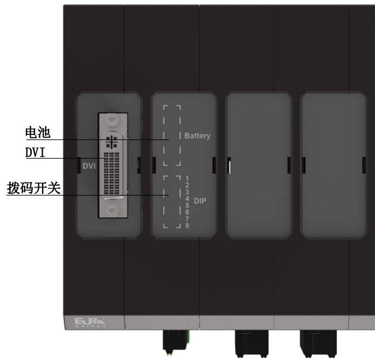
运动控制器整体视图及结构名称
