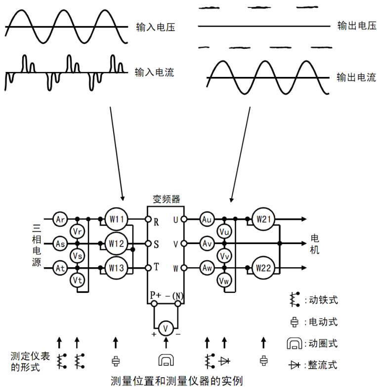
图 4-13 测量示意图
