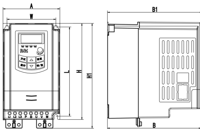
塑壳外形
