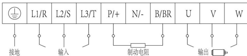
图 4-5 端子示意图
