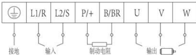
图 3-2 端子示意图
