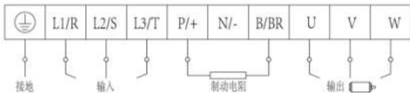
图 3-4 端子示意图
