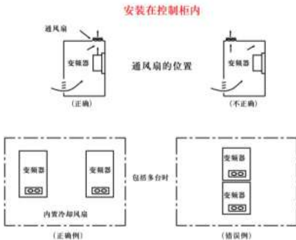
图 1-7 变频器安装在控制柜内示意图
