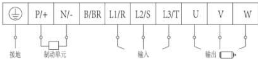
图 3-5 端子示意图
