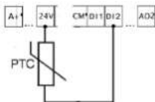
图 6-8 PTC 保护示意图
