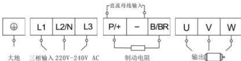
图 4-3 端子示意图
