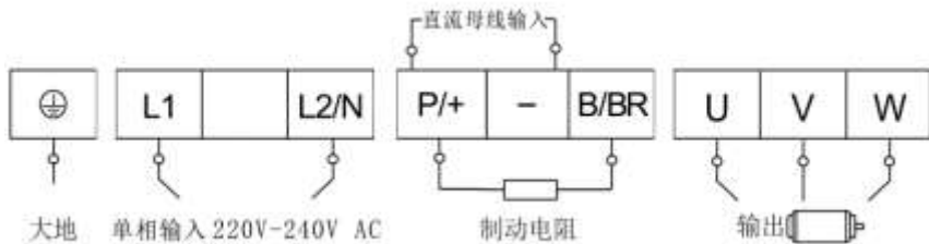
图 4-2 端子示意图
