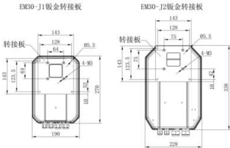
图 2-7 钣金转接板尺寸图
