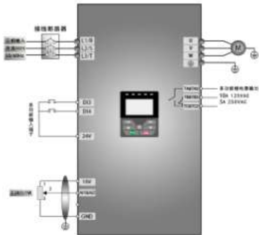
图 5-3 接线图 3
