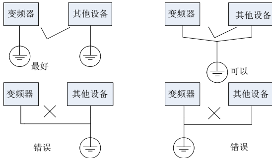
图 4-16 接地示意图
