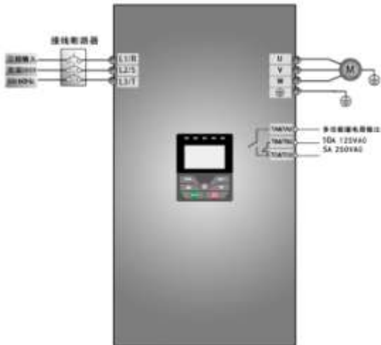
图 5-1 接线图 1
