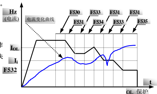
图 9-3 失速调节
