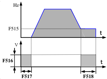
图 9-2 直流制动
