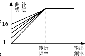
图 9-1 转矩提升曲线
