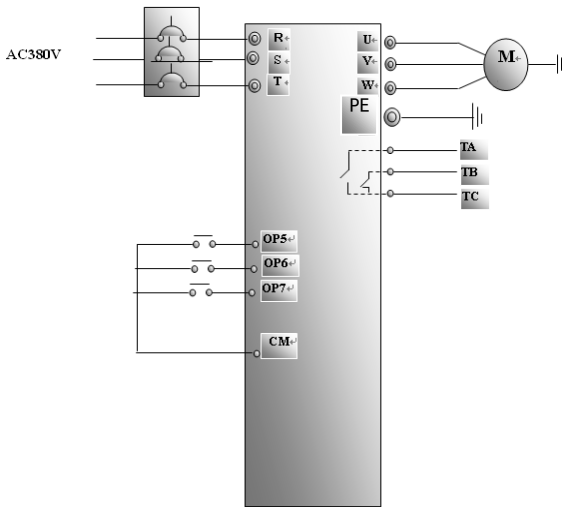
图 4-2 接线图 2
